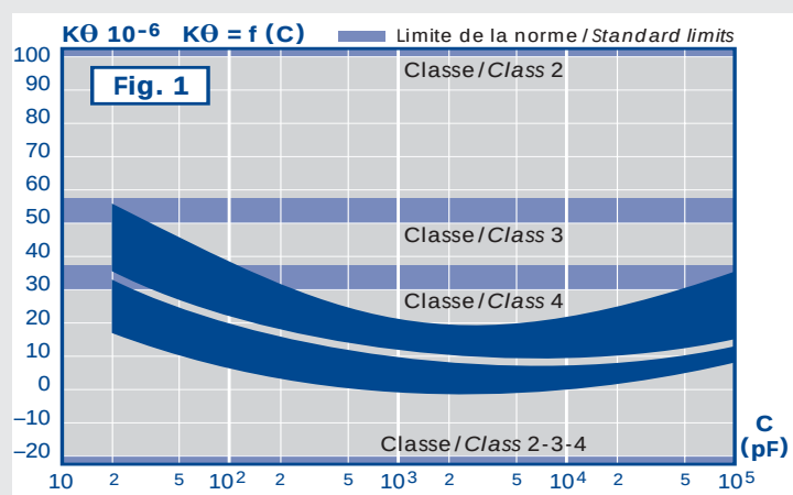
Evolution du coefficient de température en fonction de la capacité (valeur typique) Temperature coefficient versus capacitance (typical value)
